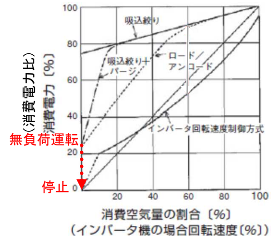
コンプレッサー制御方式と消費電力
