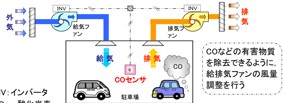
地下駐車場換気設備(例)
