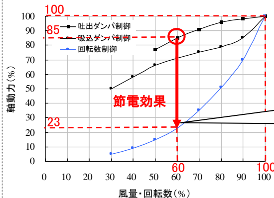
各種風量制御方式の消費電力特性
