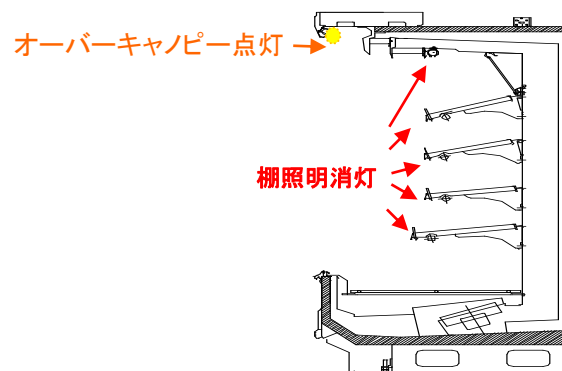
準備照明状態 (オーバーキャノピーのみ点灯)
